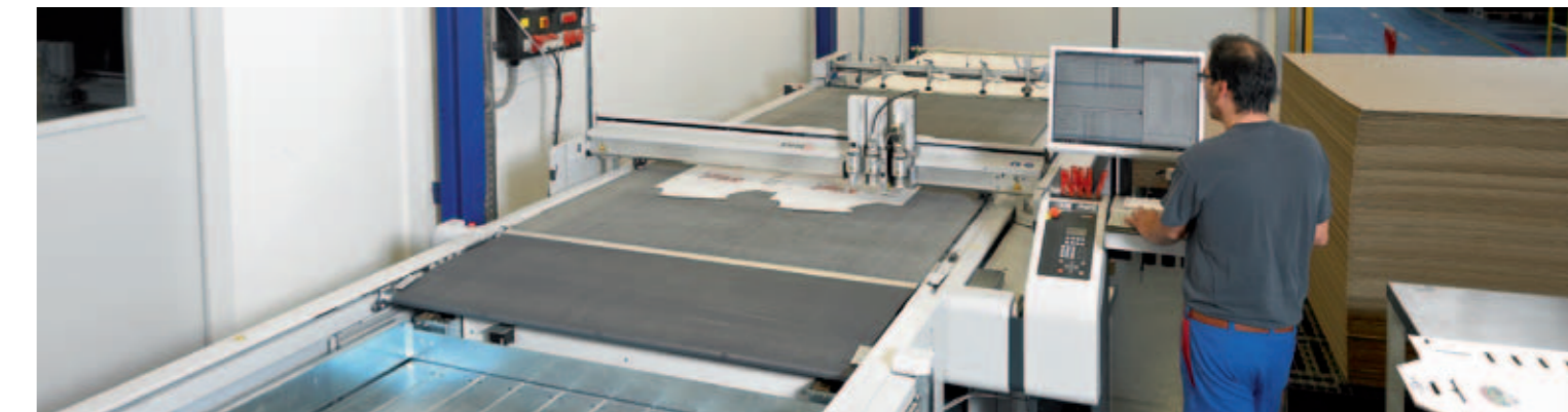
Zünd G3 L-3200 BHS Format 1800 x 3200 mm
